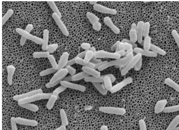
Bacilles de la tuberculose en microscopie électronique à balayage © Jean-Pierre Tissier (INRA, Villeneuve d'Ascq) et Franco Menozzi (Institut Pasteur de Lille)
